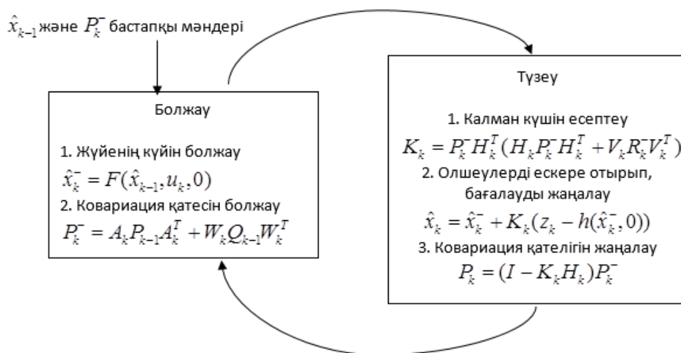
Сурет 2 - Кеңейтілген Калман фильтрінің алгоритмі
