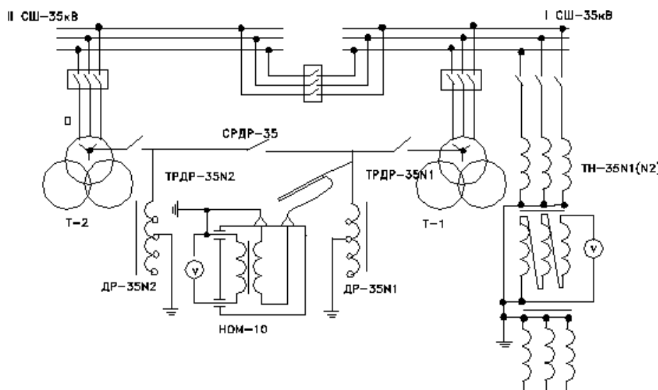
Рисунок 3— Схема замера напряжения несимметрии U_{nc} и напряжения смещения U_0 в нейтрали 35кВ силового трансформатора и замера напряжения несимметрии в разомкнутом треугольнике ЗНОМ-35 при пофазном подключении конденсатора ФМ-100 в ячейку ЗНОМ-35 на ПС 110/35/10 кВ "Камышное"
